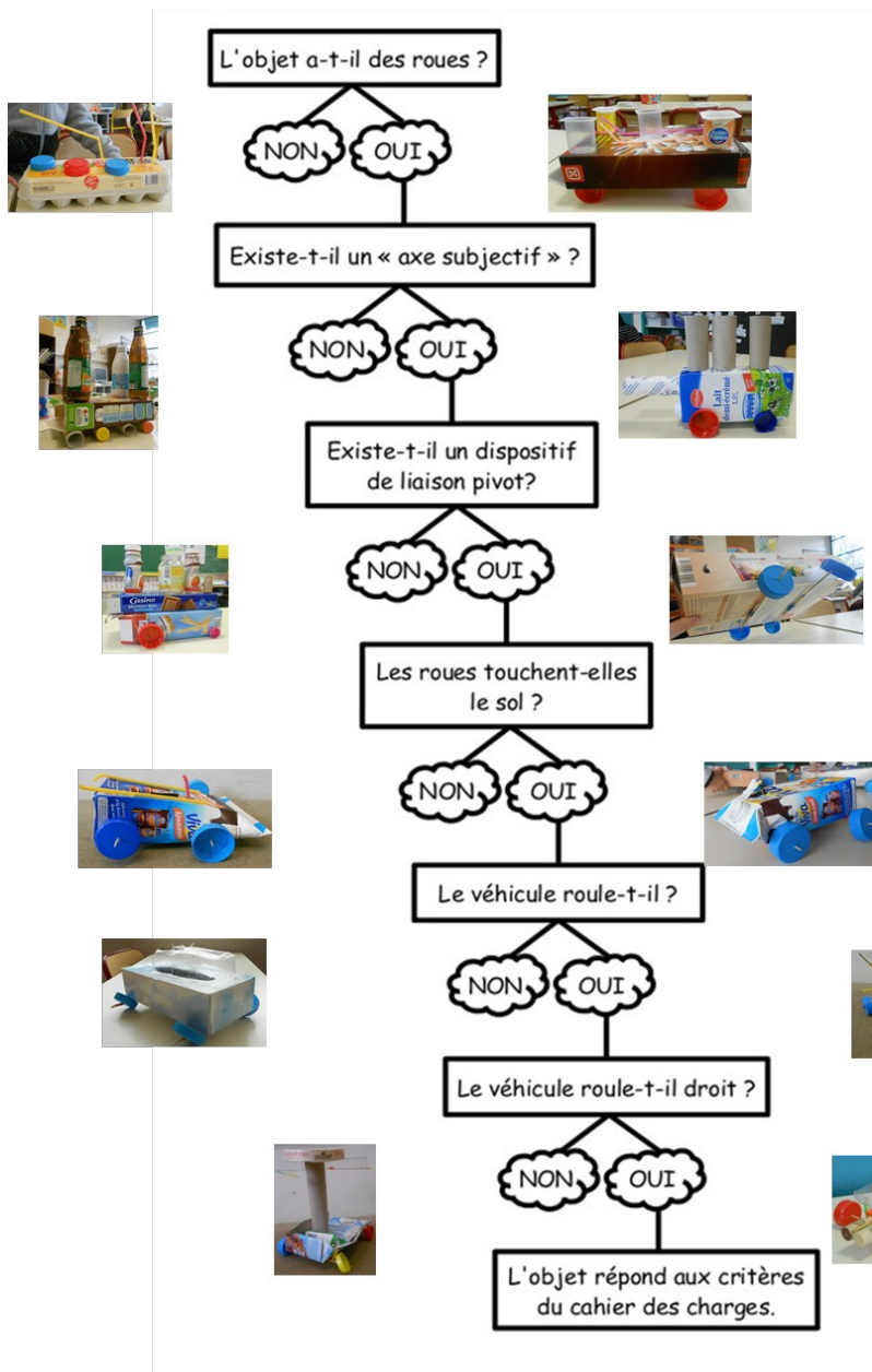
Figure 2 : Arbre d'analyse.
