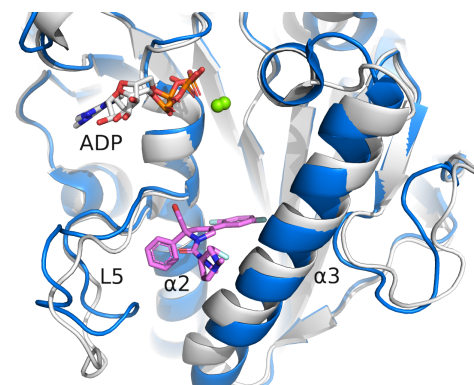
MK-0731
