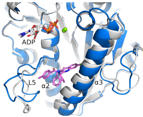
Ispinesib
