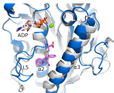
STLC
