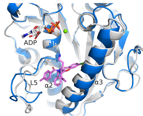
SB743921
