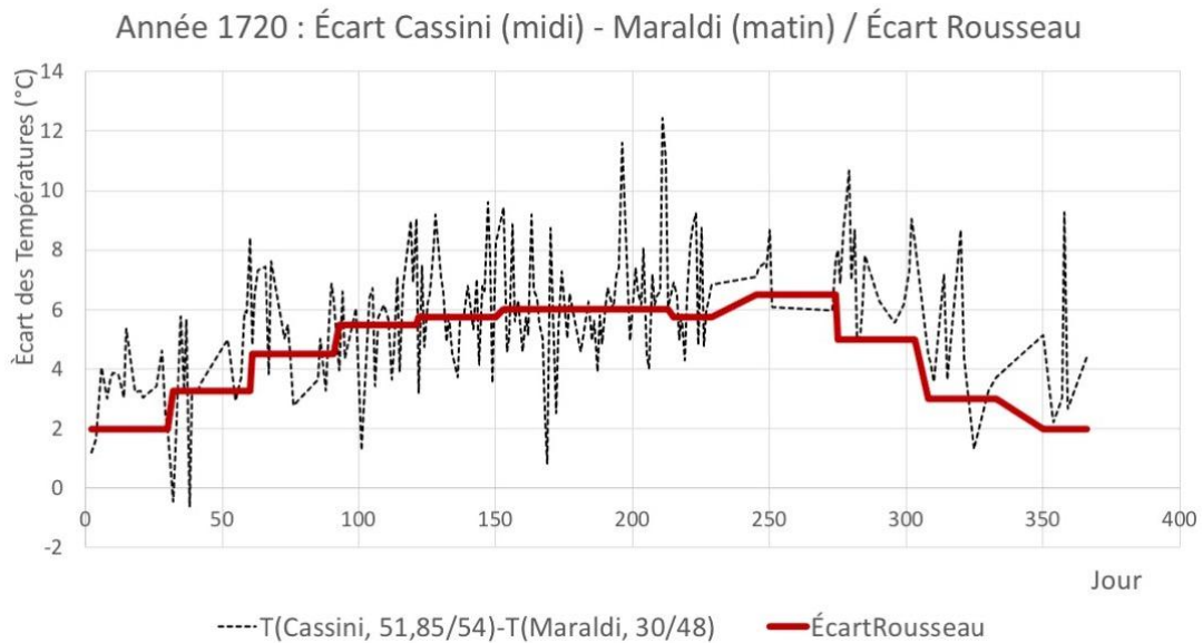
Figure 7 : Amplitude de la variation de la température entre le matin (6h-7h) et le midi à partir des mesures faites par, respectivement, Jacques Cassini (D4/2) et Jacques Philippe Maraldi (D2/22), comparée à la séquence typique fournie par Daniel Rousseau.
