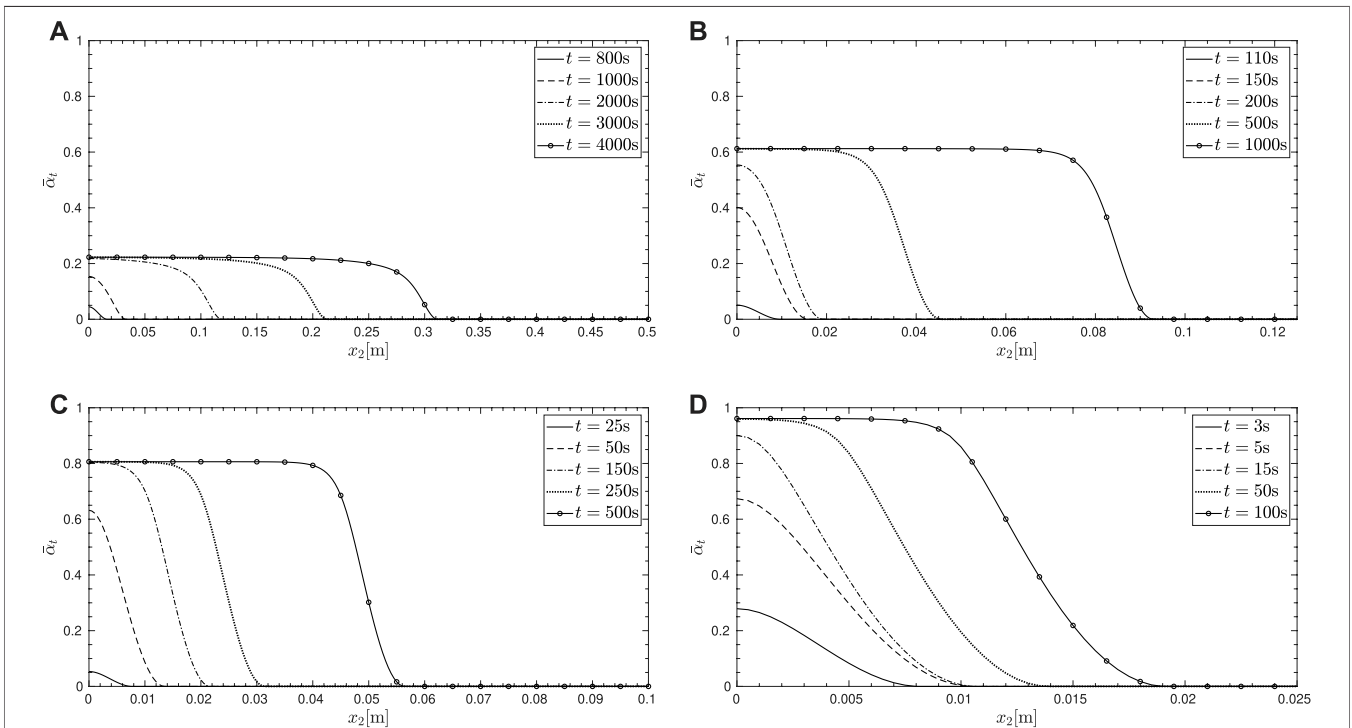
FIGURE 6 | Evolution of damage for values of w_1 (A) 2000 \text{ N}\cdot\text{m}^{-3} , (B) 1000 \text{ N}\cdot\text{m}^{-3} , (C) 500 \text{ N}\cdot\text{m}^{-3} , and (D) 100 \text{ N}\cdot\text{m}^{-3} .
