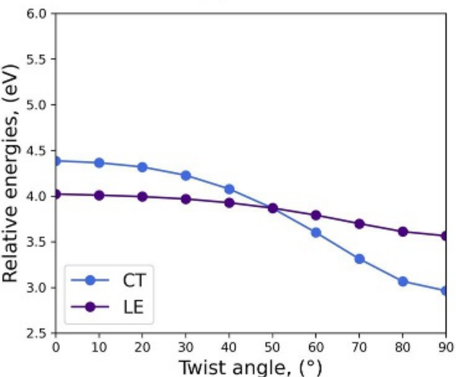
(b) CCSD
