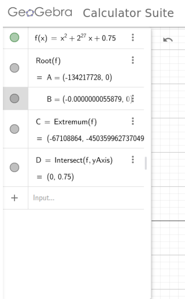
FIGURE 43 : Étude de la fonction f(x) = x^2 + 2^{27}x + \frac{3}{4} dans GeoGebra.
