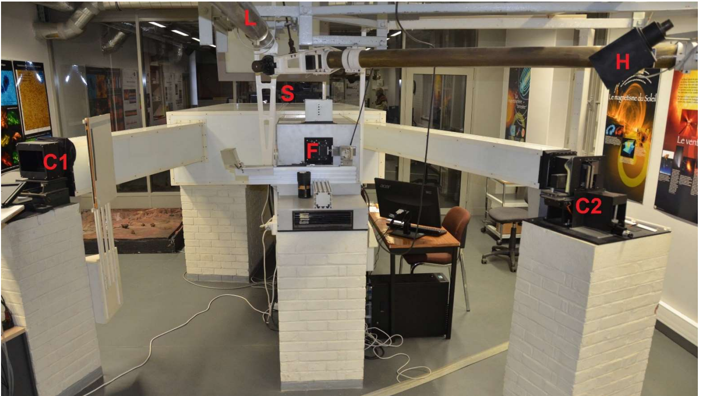
Figure 1. Spectrohéliographe de Meudon. C1 et C2 : anciennes chambres photographiques de 3.0 m pour Call K et H \alpha . S : spectrographe (contient la chambre CCD de 0.4 m, le réseau et le collimateur de 1.3 m). H = spectrohélioscope visuel escamotable à prismes rotatifs. L = porte lune de densité 1 couplé à l'objectif. F : fente du spectrographe (soleil de 37.2 mm).
