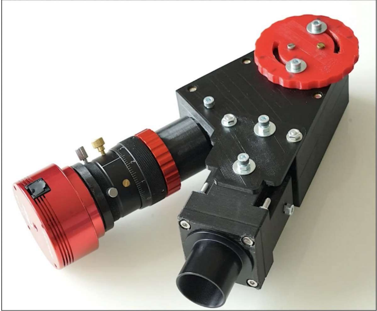
Figure 3. Vue de l'instrument Sol'Ex. On aperçoit en bas à gauche l'interface vers une lunette ou un télescope astronomique. La manette de couleur rouge permet d'orienter le réseau à diffraction et sélectionner ainsi la longueur d'onde de travail. La caméra est un modèle CMOS d'origine ZWO.
