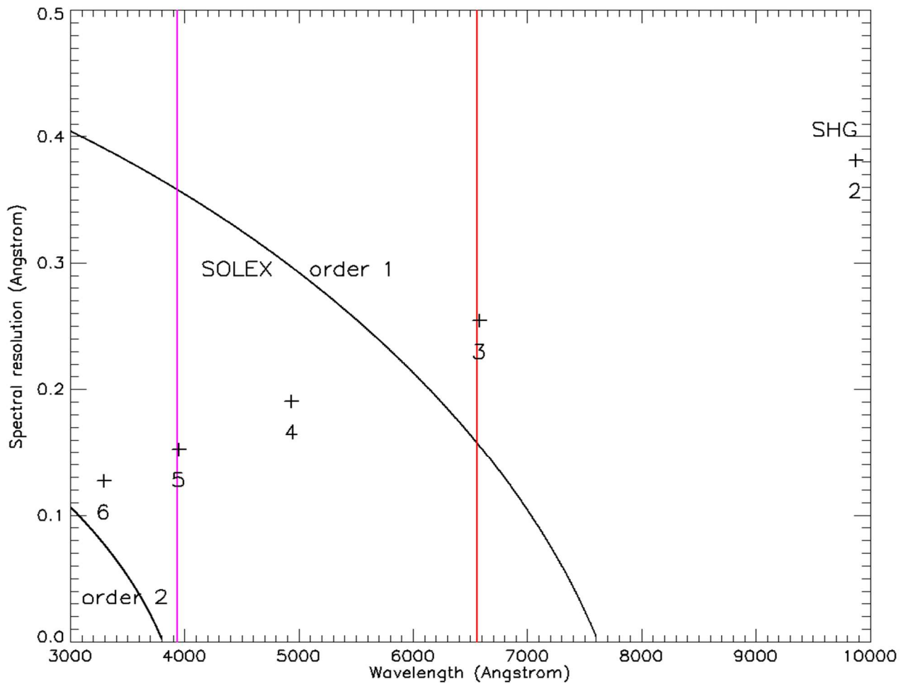
Figure 9. Résolution spectrale de Sol'Ex en Angström et comparaison avec le spectrohéliographe de Meudon fonctionnant dans les ordres 3 et 5 (2 à 6 représentés). Les comportements sont différents : pour Sol'Ex, la résolution se dégrade vers le bleu, pour Meudon elle se dégrade vers le rouge. Les résolutions spectrales des deux instruments sont dans le même ordre de grandeur, dans la gamme 0.15 - 0.30 Å. La position des raies Call K et H \alpha est indiquée par les barres (violette et rouge).
