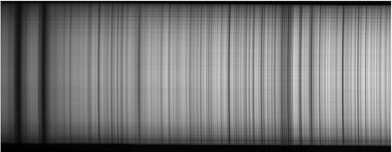
Figure 5. Exemple de spectres obtenus avec Sol'Ex : CaII K (3934 Å) et H (3968 Å), H \delta (4101 Å), CaI (4227 Å), bande moléculaire CH (4305 Å), deux raies du FeI, H \gamma (4340 Å). Longueur d'onde = axe X. La fente (axe Y) couvre ici la totalité du diamètre solaire.
