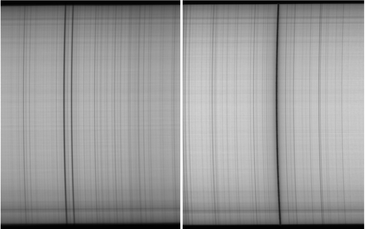
Figure 4. Exemple de spectres obtenus avec Sol'Ex : Sodium D2 (5890 Å) et D1 (5896 Å), H \alpha (6563 Å). Longueur d'onde = axe X. La fente (axe Y) couvre ici la totalité du diamètre solaire.
