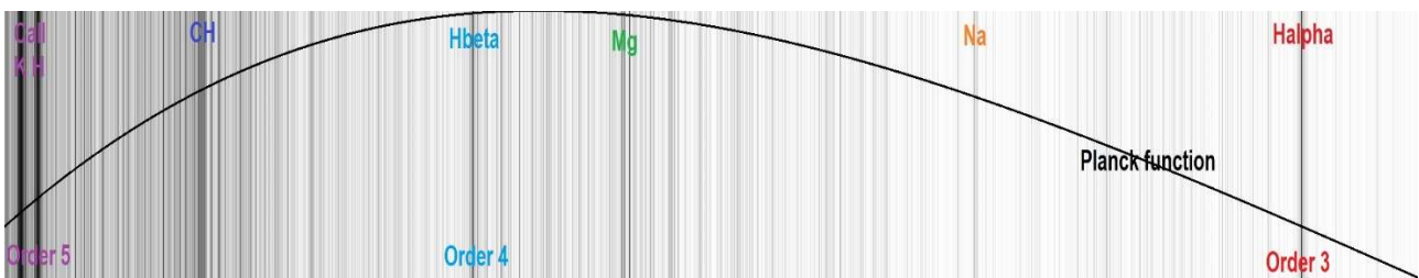
Figure 2. Spectre montrant les raies les plus aisément observables avec Sol'Ex. Toutes les raies de Fraunhofer (Call H, K violettes, série de Balmer de l'Hydrogène, Sodium D1 et D2, Helium D3, triplet du magnésium) sont observables, et bien d'autres raies photosphériques, comme celles du fer, sensibles à l'effet Zeeman qui est mesurable avec Sol'Ex en y adjoignant un analyseur de polarisation circulaire. Le spectrohéliographe de Meudon ne permet d'observer que dans les ordres 3, 4 et 5 indiqués.
