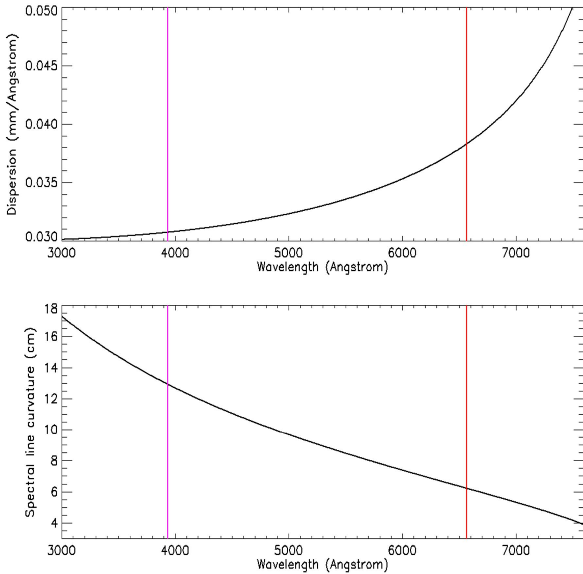
Figure 8. Dispersion de Sol'Ex en mm/Angström (en haut) et rayon de courbure des raies en cm (en bas), en fonction de la longueur d'onde d'observation. Les raies sont courbes sur le détecteur et la courbure est corrigée par le programme de traitement INTI. La position des raies Call K et H \alpha est indiquée par les barres (violette et rouge).
