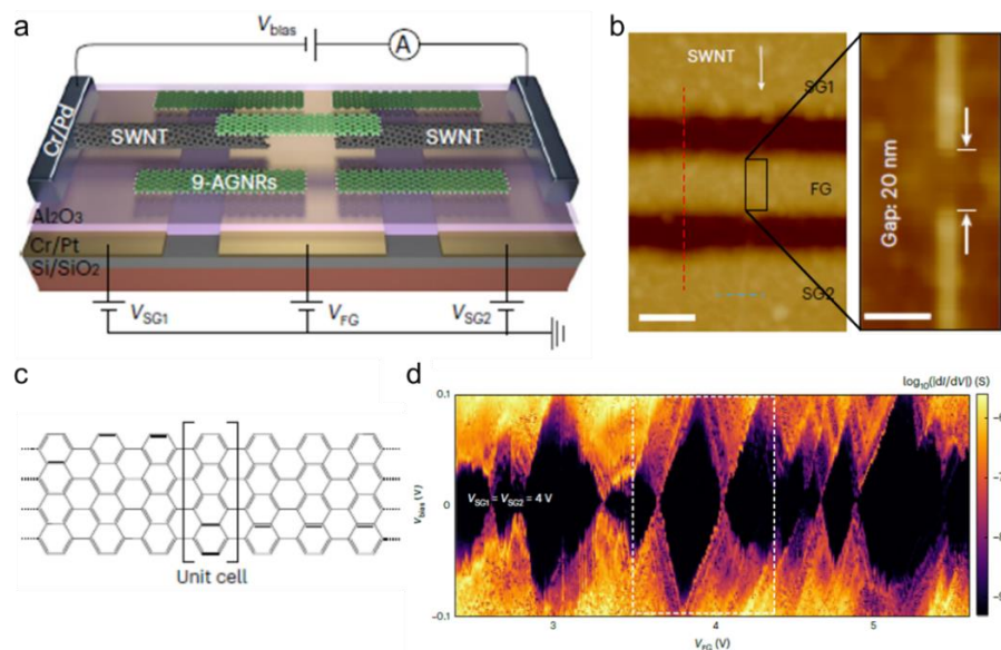
Figure 3 : (a) Schéma du transistor avec le circuit de mesure ; (b) Image AFM des trois grilles notées SG1, FG et SG2 sous le nanotube de carbone à simple paroi, avec un zoom sur le nanogap réalisé dans le nanotube pour accueillir de nanoruban (barre d'échelle de 20 nm) ; (c) Structure moléculaire du nanoruban de graphène nommé 9-AGNR étudié ; (d) Transport électronique dans les transistors de 9-AGNR avec des électrodes en nanotubes à paroi unique métalliques : la conductance différentielle est présentée en échelle de couleur en fonction de V_{FG} et V_{Bias} à V_{SG1} = V_{SG2} = 4 V. (Figure adaptée de l'article : Nature Electronics 6, pages 572–581, 2023).
