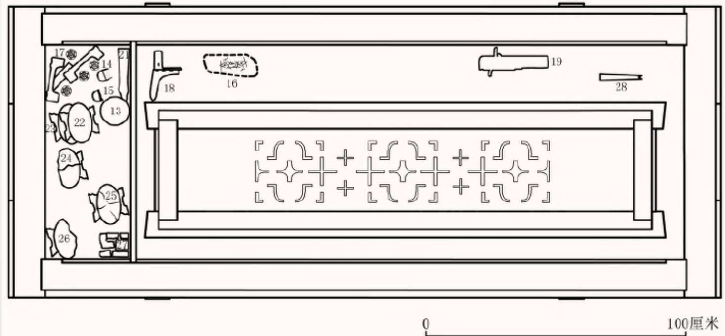
图四 M798椁室平面及随葬器物分布
