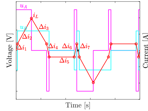
(d) DAB ZVS Triangular 2 (novel)
