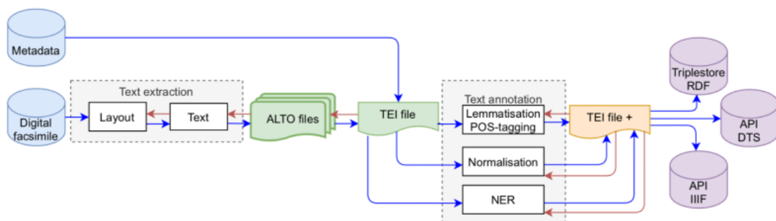
Figure 3: Chaîne de traitement des données dans le projet Gallic(orpor)a, issue d'Ariane Pinche, Kelly Christensen et Simon Gabay, « Between automatic and manual encoding Towards a generic TEI model for historical prints and manuscripts », TEI Conference and Members&apos; Meeting, Newcastle, 2022.
