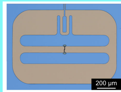
Transmon qubit 15
