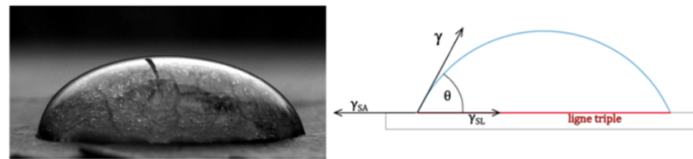
Figure 1 : Goutte sessile. (a) Photo d'une expérience ; (b) modèle de Young pour les forces à la ligne de contact [1].
