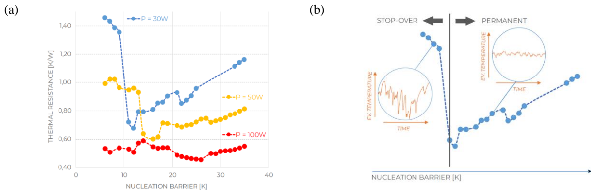
Fig. 1 Simulations CASCO d'un caloduc : (a) étude de performance d'un caloduc oscillant en fonction de la barrière de nucléation pour plusieurs niveaux de puissance P de l'évaporateur et T_{cond}=20^{\circ}C . (b) Variation de la température de l'évaporateur dans les régimes des oscillations intermittentes (stop-over) et permanentes.
