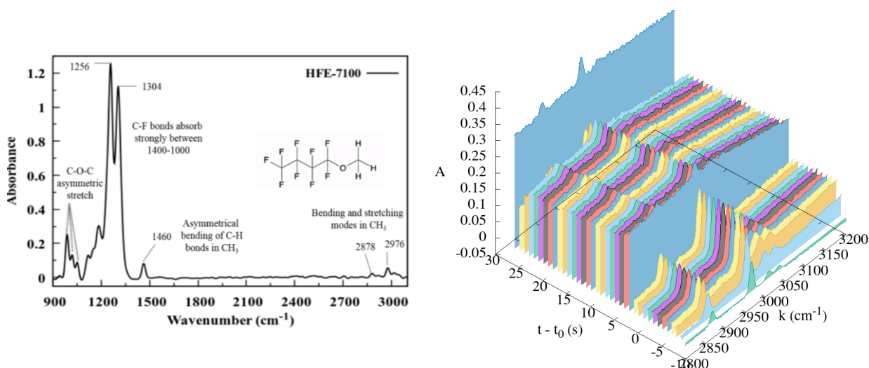
Figure 2 : Gauche : Spectre FT-IR du HFE7100. Droite : Spectre FT-IR obtenu lors d'une parabole dans la gamme 2800,3200 \text{cm}^{-1} (parabole P26, résolution 4 \text{cm}^{-1} , 1 Hz). t_0 est le temps auquel survient la détente créant l'aérosol. La ligne de base est obtenue à partir d'un spectre de référence d'air propre.
