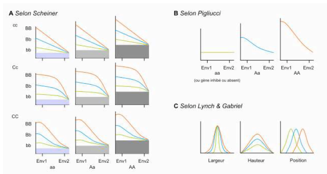
Figure 1 - Définitions des gènes de plasticité illustrées à l'aide de normes de réaction d'un trait (en ordonnée) en fonction de l'environnement (en abscisse). (A) La conception de Scheiner (1993) est la plus complexe avec trois types de gènes à deux allèles : il y a des gènes qui codent pour la valeur moyenne du trait (gène A dont l'effet est symbolisé par les rectangles grisés), d'autres pour la pente (gène B) et d'autres pour la forme (gène C). (B) Selon Pigliucci (1996), les gènes de plasticité sont des gènes de régulation qui répondent directement aux stimuli environnementaux. Dans le cas où le gène est absent, inhibé ou homozygote récessif, le phénotype ne change pas. (C) Lynch & Gabriel (1987) proposent un système à trois gènes influençant respectivement la largeur, la hauteur et la position des normes de réaction de forme gaussienne. Figure tirée de Foray (2011) reproduite et modifiée de Windig et al. 2004.
