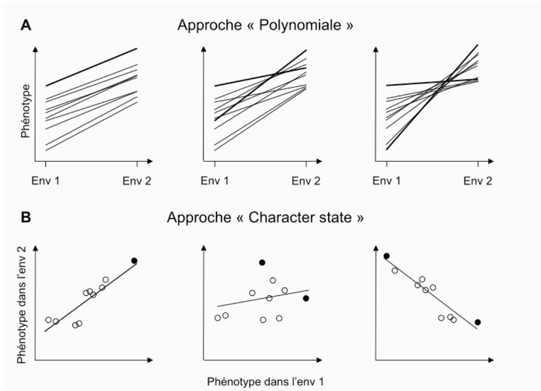
Figure 3 - Deux principaux modèles de génétique quantitative utilisés pour étudier les normes de réaction. On considère 10 génotypes dans deux environnements. Dans l'approche « polynomiale », la valeur phénotypique des génotypes est indiquée en fonction de la valeur de l'environnement alors que dans l'approche « character state », la valeur phénotypique d'un génotype dans un environnement est exprimée en fonction de sa valeur dans un autre environnement. Trois types d'interactions génotype-environnement sont représentés selon que les hiérarchies entre génotypes dans les deux environnements sont (i) globalement les mêmes, (ii) indépendantes, (iii) globalement inversées (trade-off environnemental). Les génotypes présentant un optimum dans au moins l'un des deux environnements sont figurés en gras. Figure tirée de Ris 2003.
