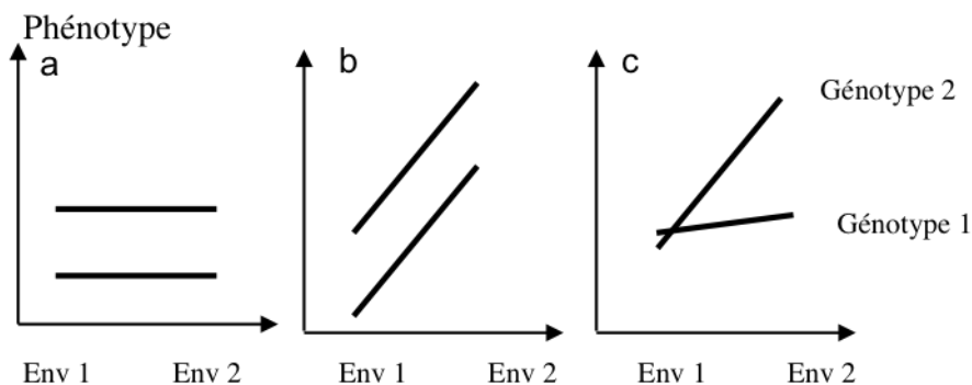
Figure 2- Indépendance des concepts de variation génétique (VG), plasticité phénotypique (PP) et variation génétique de la plasticité phénotypique (VPP). a) VG existe mais il n'y a pas de PP et de VPP. b) il existe de la VG et de la PP mais pas de VPP. c) VG, PP et VPP sont significatifs. (D'après Pigliucci 2001).
