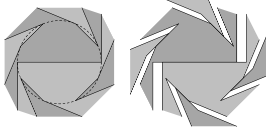
FIGURE 4. Régions bordées par des plans croches, et leurs translâtées (coupe horizontale). Le cercle est une carte affine de \mathbb{H}^2 .
