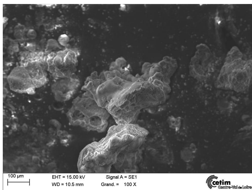
FIGURE IV.2.5 – Vue générale des produits de combustion solides obtenue par MEB
