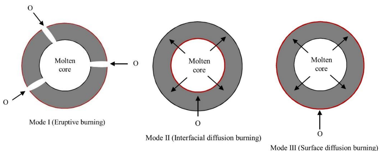
FIGURE II.2.1 – Schématisation des différents modes d'oxydation possibles durant la phase d'allumage d'une particule d'aluminium (Sundaram, 2016)
