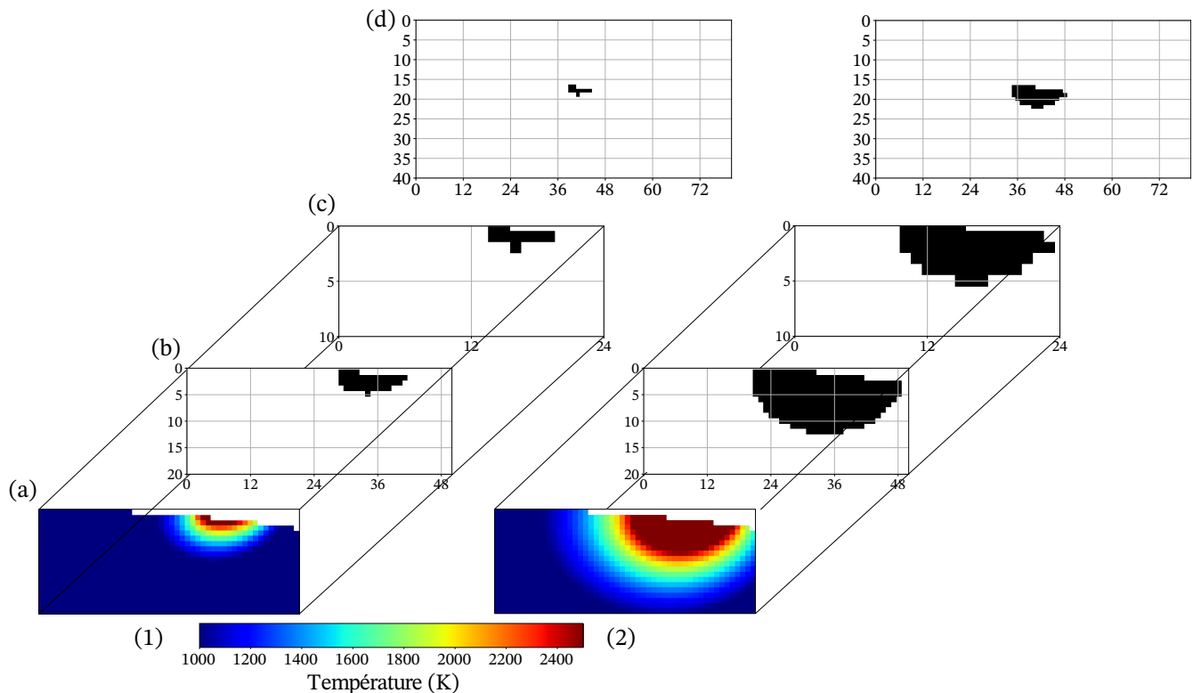
FIGURE 4.15: Processus de binarisation des images : (1) P_{laser} = 350\text{ W} et V_{laser} = 5\text{ mm}^{-1} . (2) P_{laser} = 650\text{ W} et V_{laser} = 1\text{ mm}^{-1} . (a) Résultat des simulations thermiques (en y = 0 ). (b) Identification de la zone fondue ( T > 1673\text{ K} ). (c) Ajustement des dimensions de l'image pour correspondre aux caractéristiques du détecteur de rayons X. (d) Ajustement des dimensions de l'image ( 40 \times 80\text{ px} )
